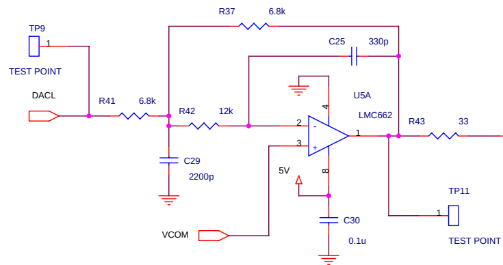
LPF( f_c 20\text{kHz} )
