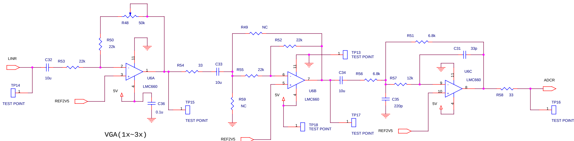
LPF( f_c 200\text{kHz} )
