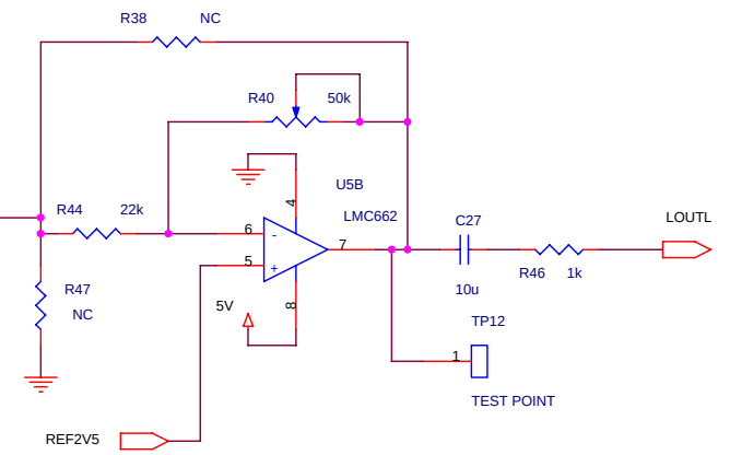
VGA( 0x \sim 2x , can be LPF/HPF)
