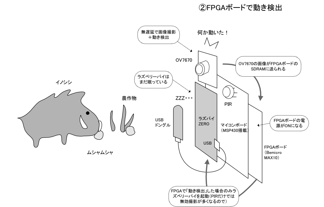
図2 電源ONですぐ動くFPGA+ネット接続できるラズベリーパイのコラボレーション！
