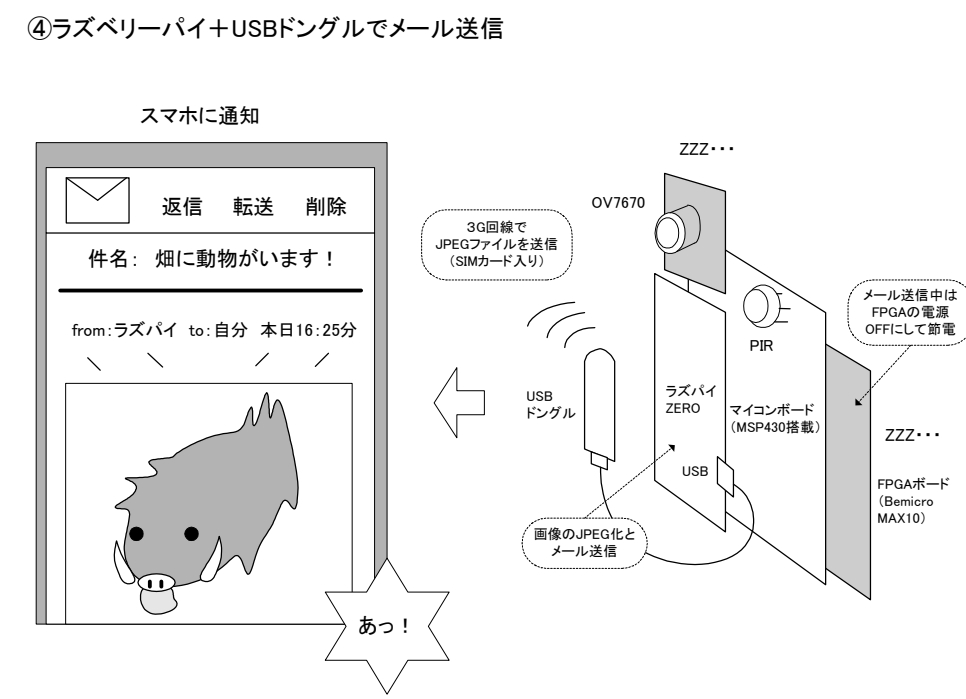
図2 電源ONですぐ動くFPGA+ネット接続できるラズベリーパイのコラボレーション！
